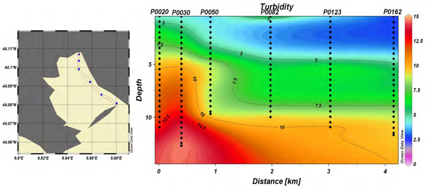
Fig.12 Parametro Torbidità (FTU) - Esempi di sezioni dei transetti T0021 (Levante) e T0022 (Ponente) interni alla diga
