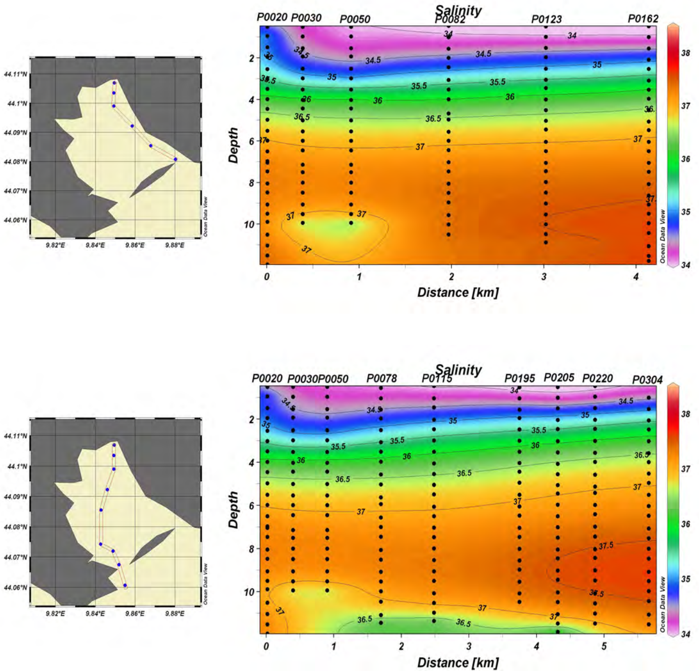
Fig.35 Parametro Salinità (PSU) - Esempi di sezioni dei transetti T0021 (Levante) e T0022 (Ponente) interni alla diga
