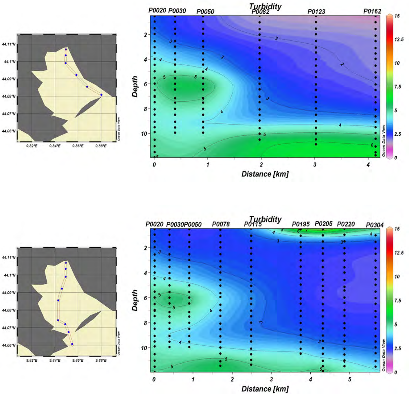
Fig.36 Parametro Torbidità (FTU) - Esempi di sezioni dei transesti T0021 (Levante) e T0022 (Ponente) interni alla diga
