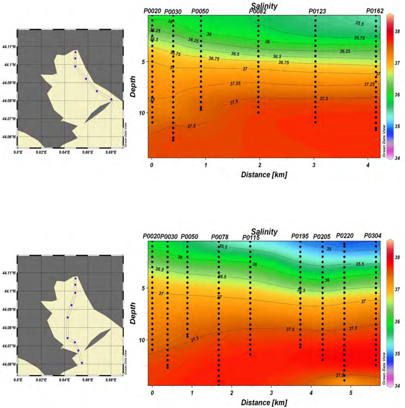
Fig.11 Parametro Salinità (PSU) - Esempi di sezioni dei transetti T0021 (Levante) e T0022 (Ponente) interni alla diga
