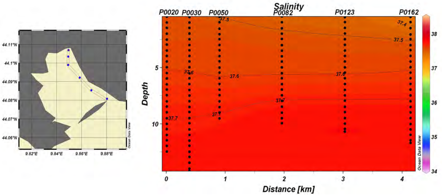
Fig.29 Parametro Salinità (PSU) - Esempi di sezioni dei transetti T0021 (Levante) e T0022 (Ponente) interni alla diga
