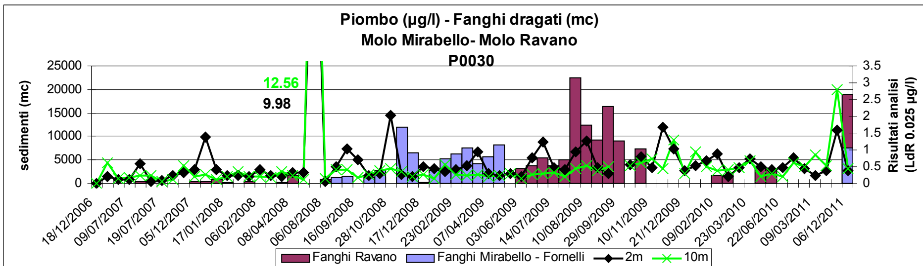
Fig.8 Andamento dei metalli: Pb, Sn, V, Zn, Hg, As eseguito nelle stazioni di campionamento P0030-P0117-P0199, a due profondità (2 m dalla superficie e +2 m dal fondo) nell'intero periodo di dragaggio (dicembre 2006-dicembre 2011)
