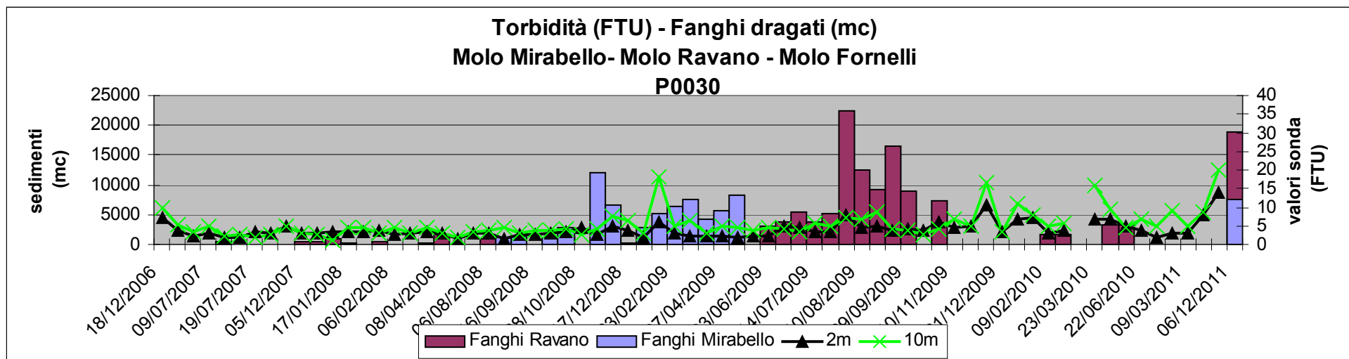
Fig.7 Andamento parametro torbidità in tre stazioni di campionamento (P0030- P0117-P0199), a due profondità (2 m dalla superficie e +2 m dal fondo) nell'intero periodo di dragaggio (dicembre 2006-dicembre 2011)
