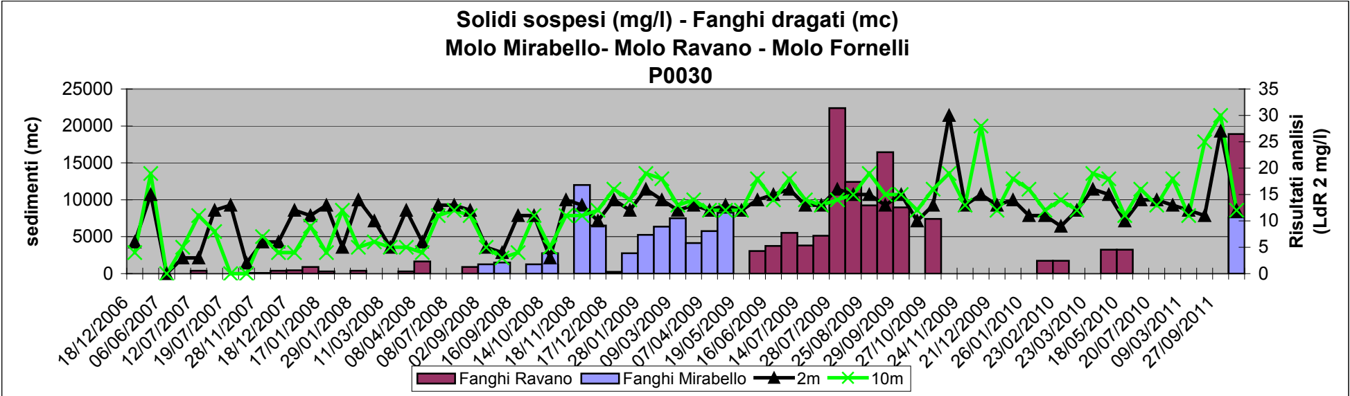
Fig.6 Andamento parametro Solidi Sospesi Totali in tre stazioni di campionamento (P0030- P0117-P0199), a due profondità (2 m dalla superficie e +2 m dal fondo) nell'intero periodo di dragaggio (dicembre 2006-dicembre 2011)
